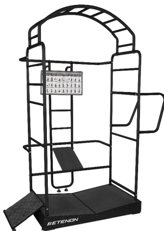
AS1602 JAULA DE ESTIRAMIENTO DIMENSIONES: L: 155 x A: 107 x Al: 228 cm. PESO TOTAL: 110 kg.
